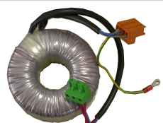
3215.02.0852V02 ECO Transformer Trasformatore ECO (127÷230V)
